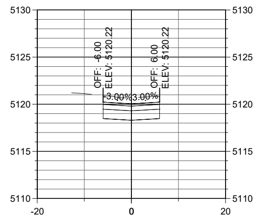
STA. 24+60
