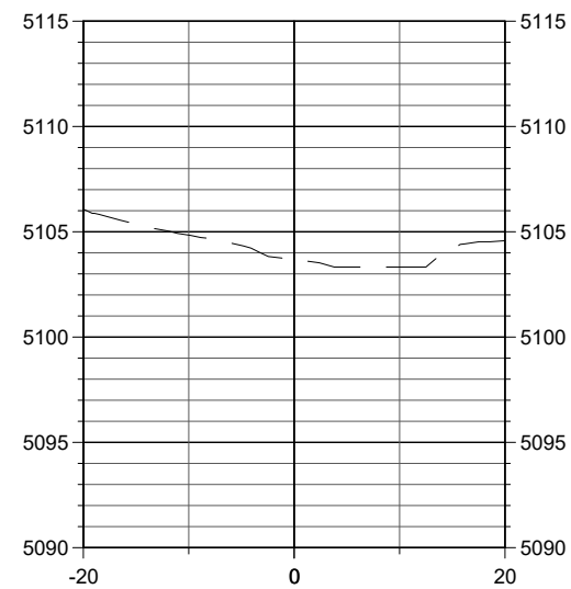
STA. 81+81
