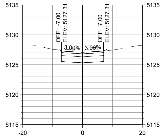
STA. 33+00
