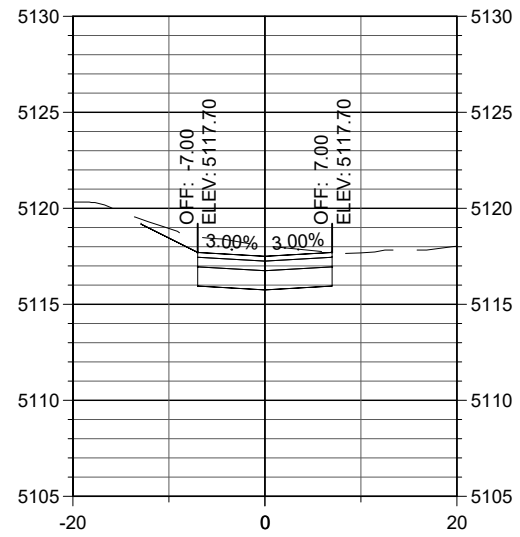
STA. 31+40
