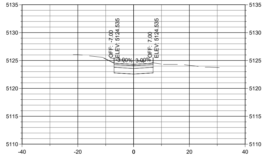
STA. 70+80
