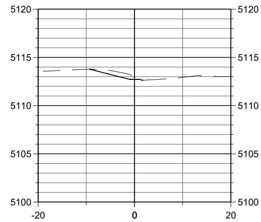
STA. 80+60
