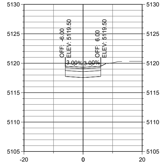
STA. 24+20
