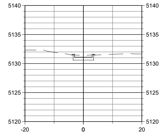
STA. 91+20
