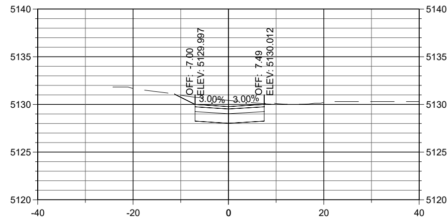
STA. 8+00
