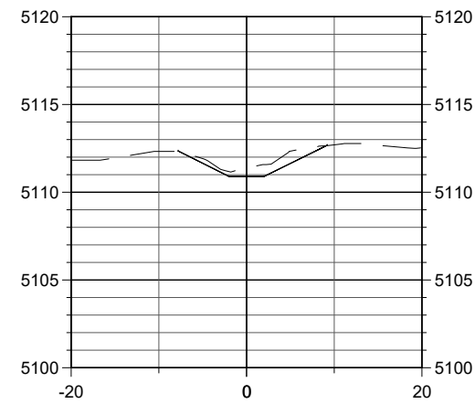
STA. 80+97
