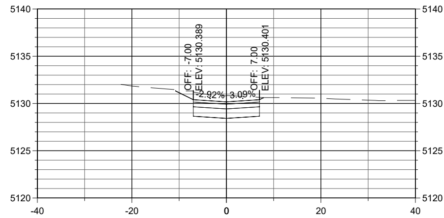
STA. 8+20
