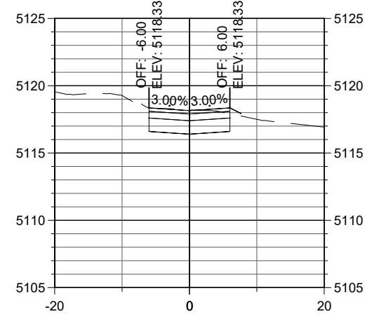
STA. 23+40
