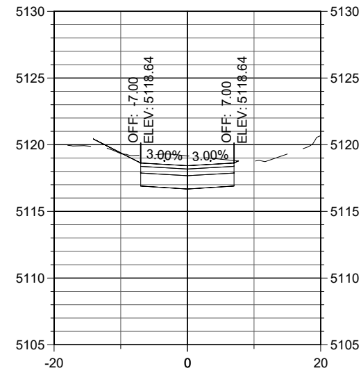
STA. 31+60
