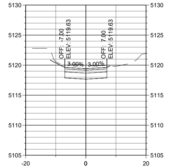
STA. 31+80
