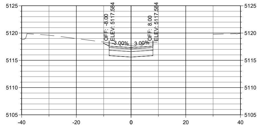
STA. 52+20
