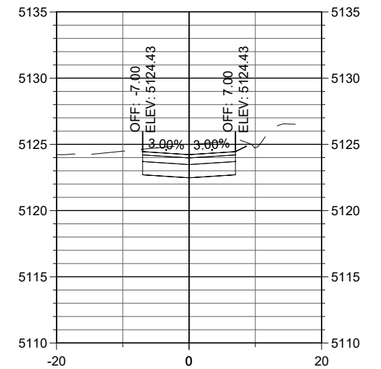
STA. 32+60
