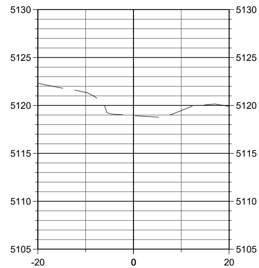
STA. 23+00
