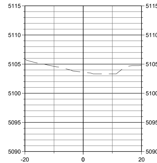
STA. 81+80
