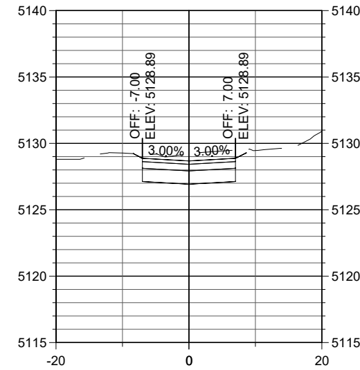
STA. 33+20
