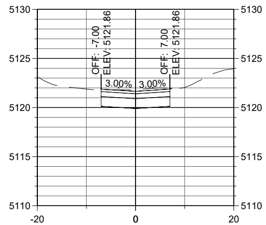
STA. 32+20
