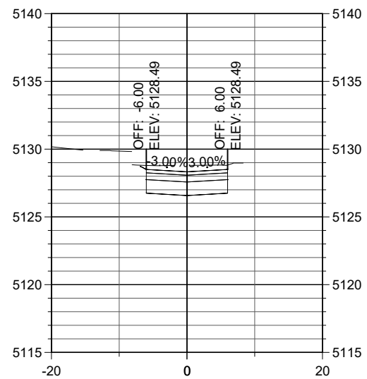
STA. 26+40
