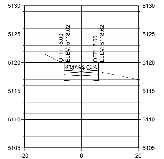
STA. 23+60
