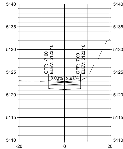
STA. 32+40
