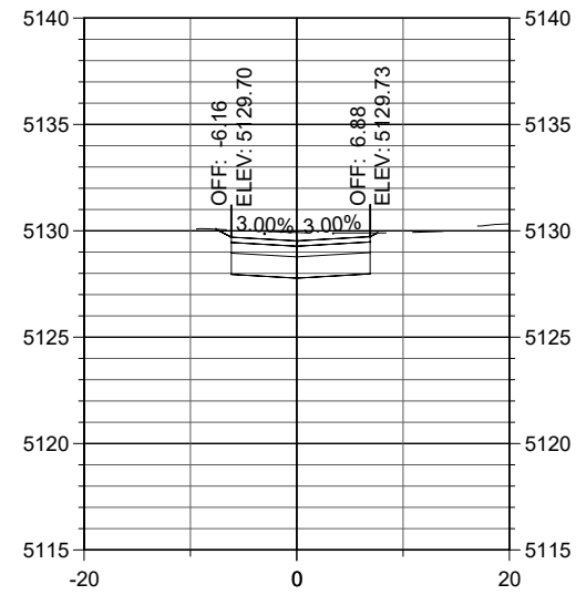
STA. 27+00
