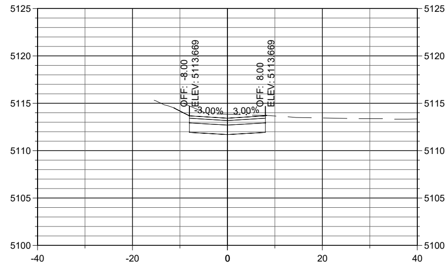
STA. 53+80
