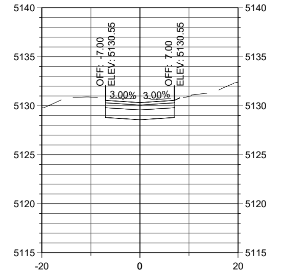
STA. 33+40
