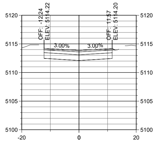
STA. 30+60
