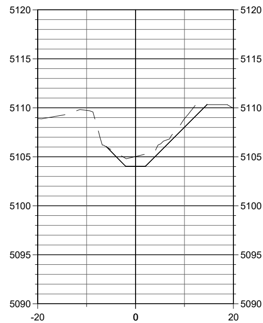
STA. 81+60
