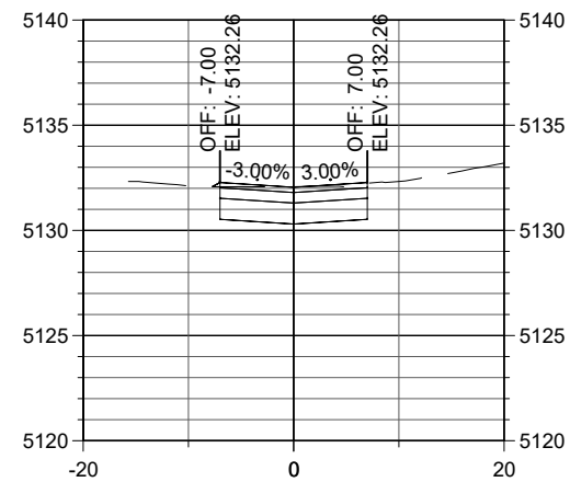
STA. 33+60
